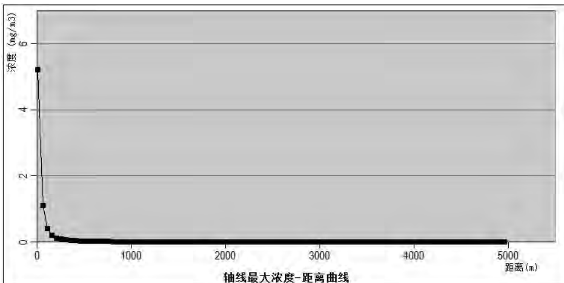
图 6.7-1 最不利气象条件下硝酸轴线最大浓度-距离曲线
