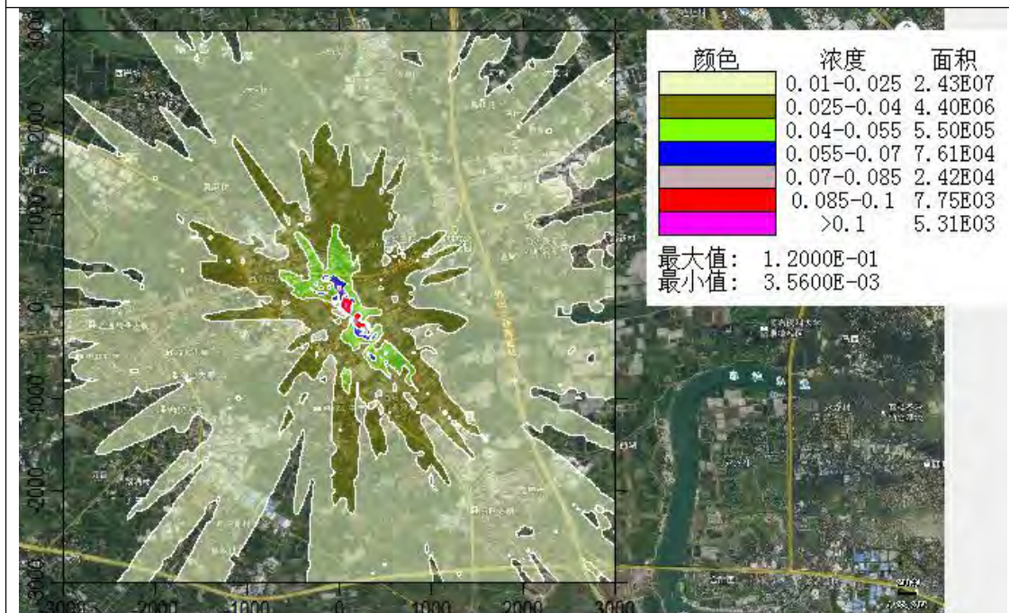
二氧化氮小时浓度贡献值分布图
