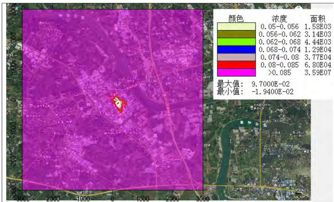
叠加现状浓度后的二氧化氮 98%日均浓度分布图
