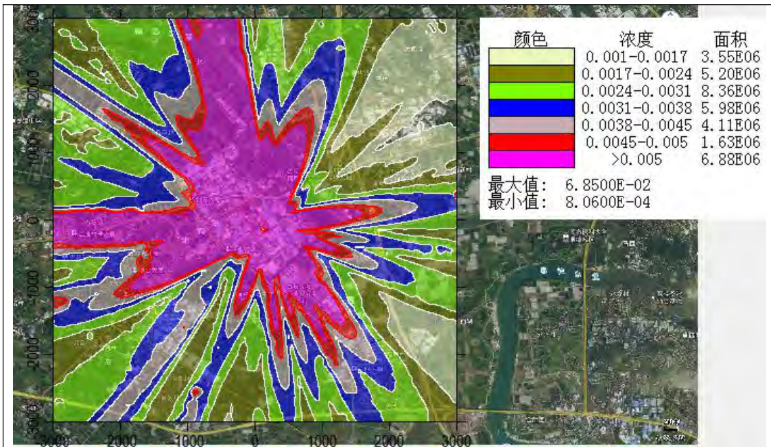
PM 10 日均浓度贡献值分布图
