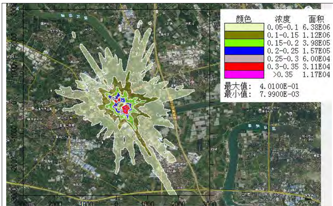
VOCs8 小时值浓度贡献值分布图
