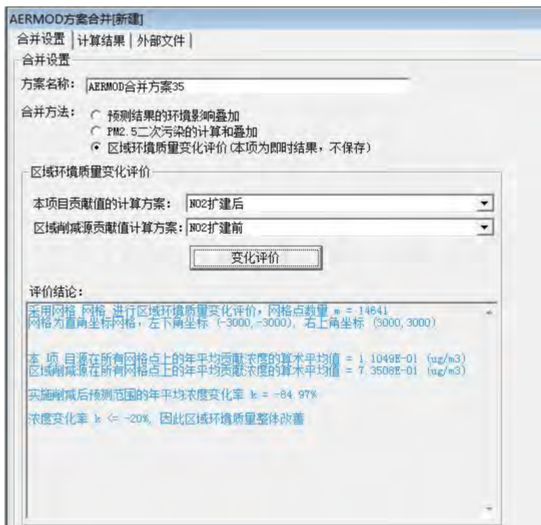
图 5.3-18 NO 2 年平均质量浓度变化预测结果
