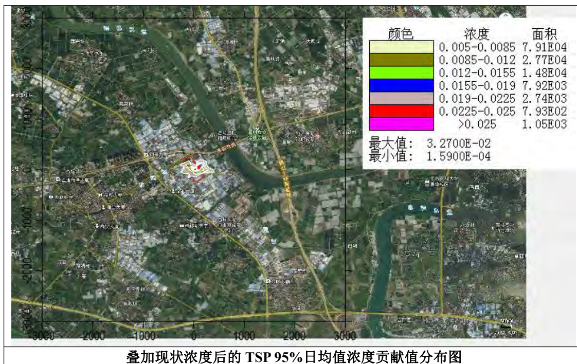
图 5.3-19 评价范围内预测因子的预测结果分布图 单位: \text{mg}/\text{m}^3
