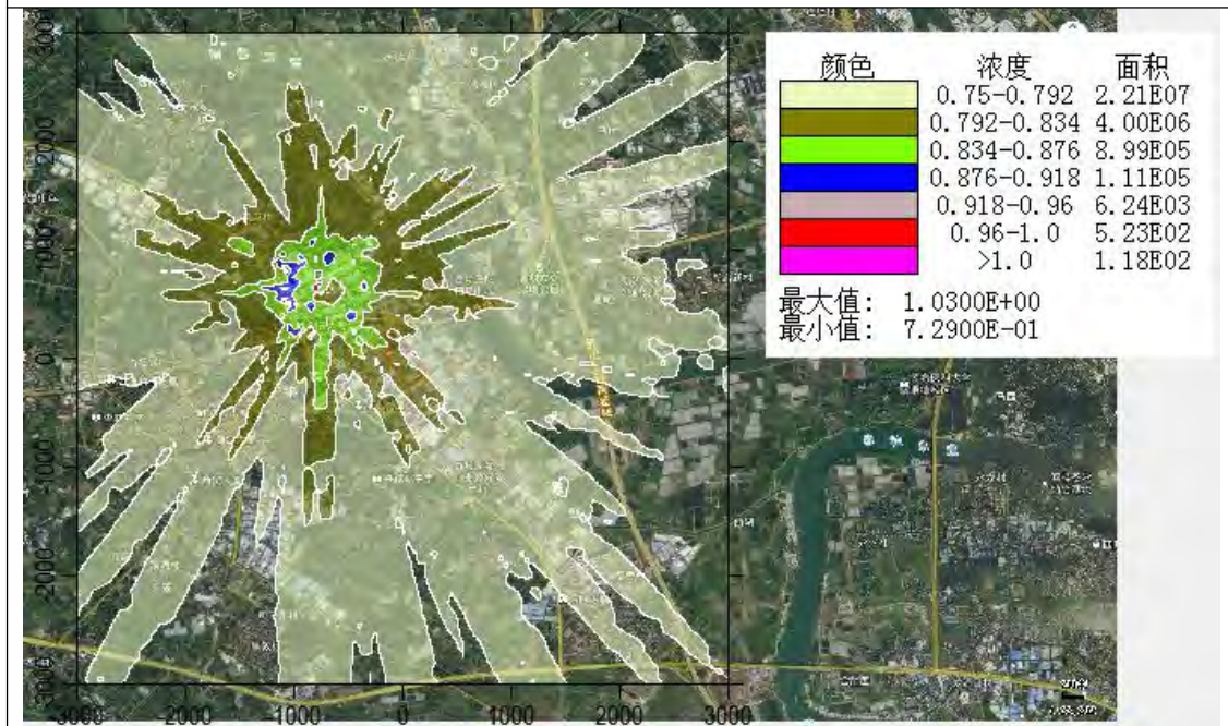
叠加现状浓度后的非甲烷总烃小时浓度分布图
