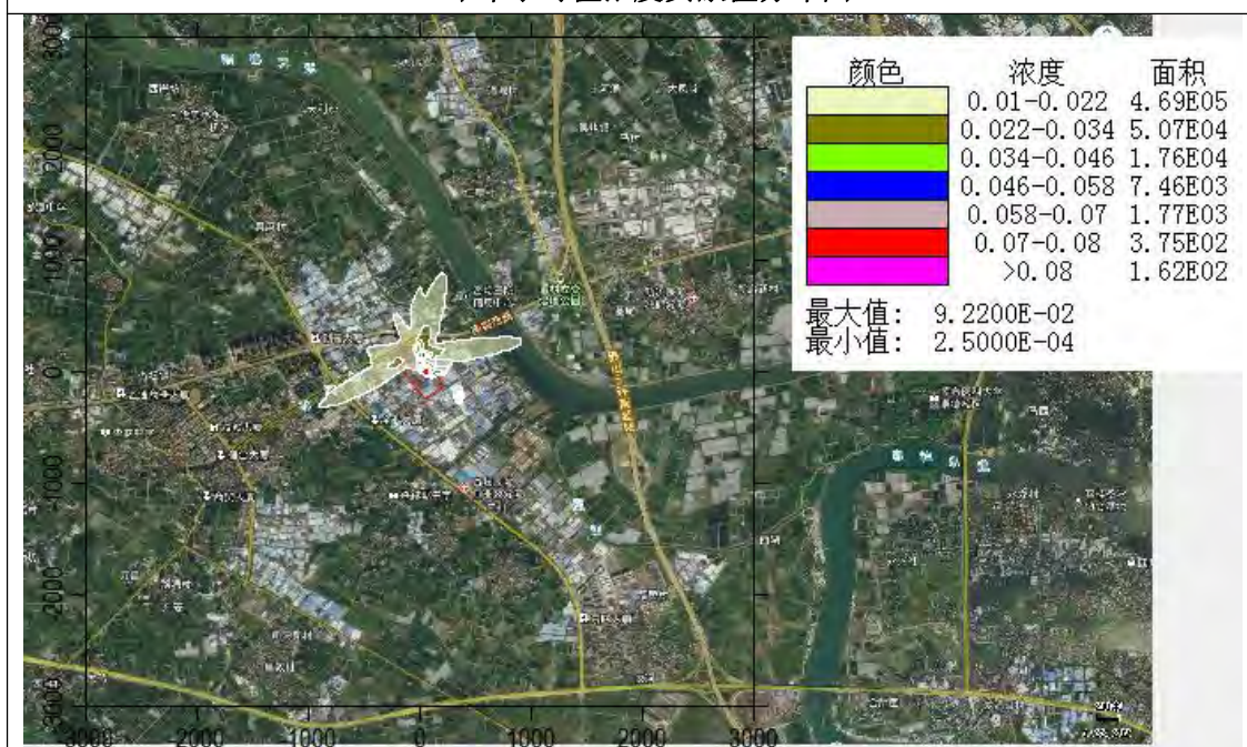
叠加现状浓度后的二甲苯小时浓度分布图
