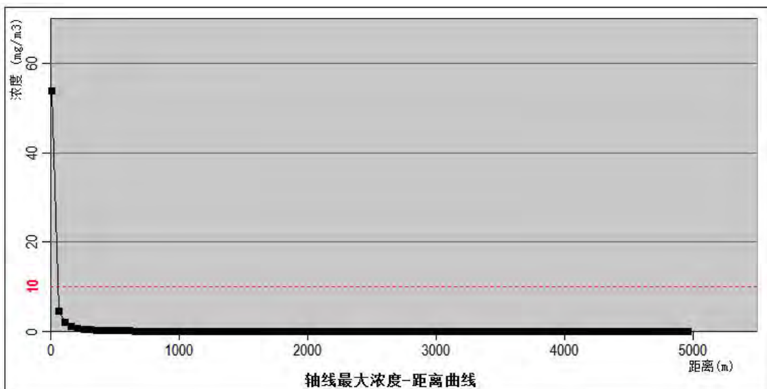
图 6.7-2 最不利气象条件下甲醇轴线最大浓度-距离曲线
