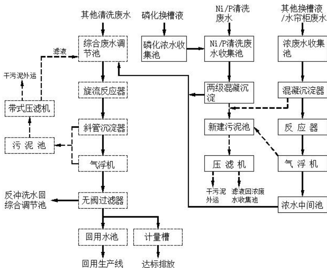
图7.1-1 废水处理工艺流程
