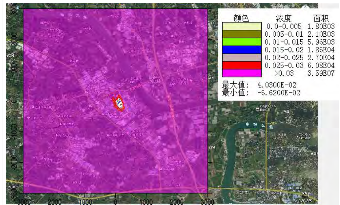
叠加现状浓度后的二氧化氮年均浓度分布图
