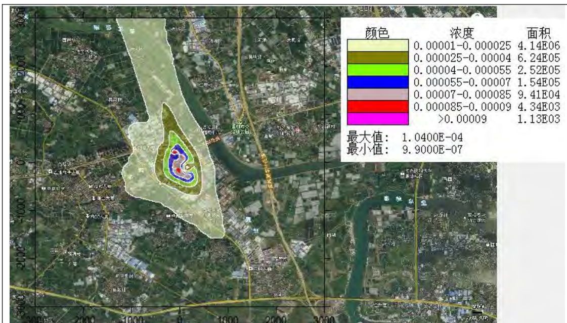
二氧化硫年均浓度贡献值分布图
