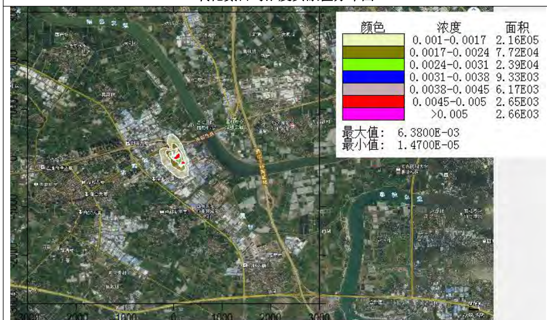
二氧化氮年均浓度贡献值分布图
