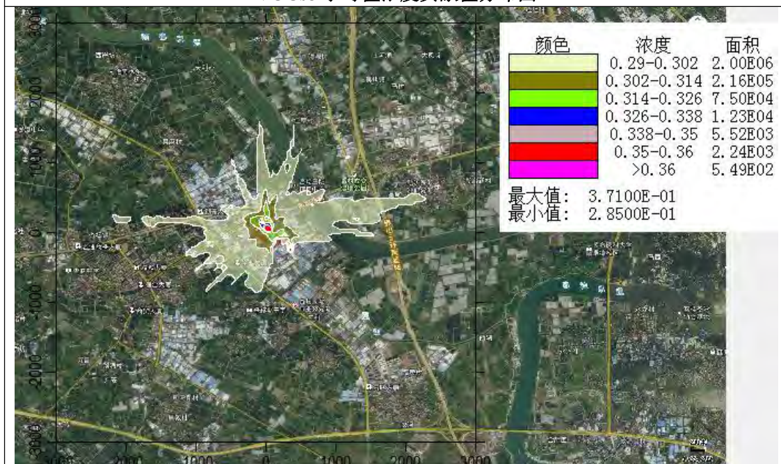
叠加现状浓度后的 VOCs8 小时浓度分布图
