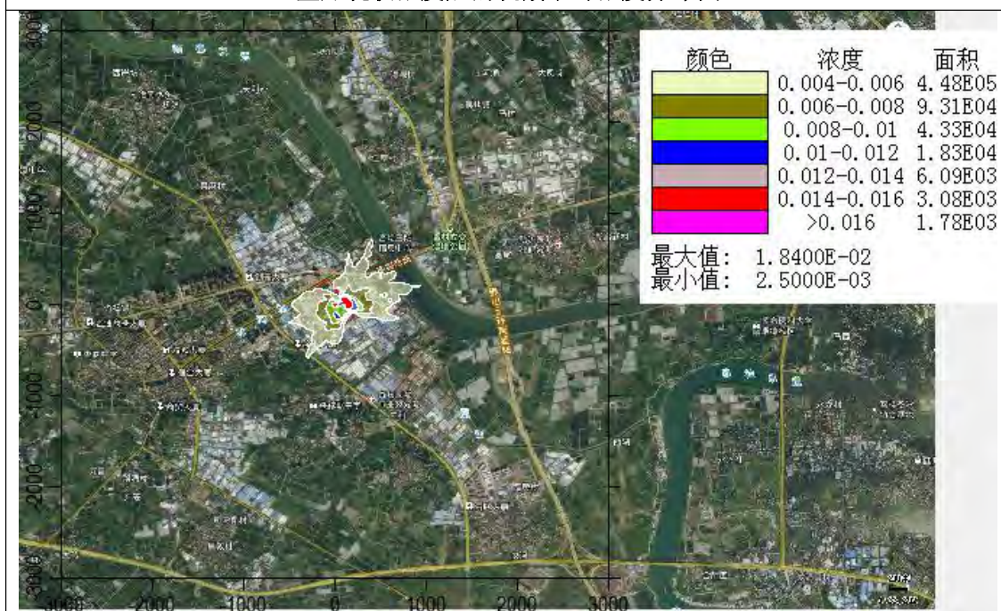
叠加现状浓度后的硫酸日均值浓度分布图
