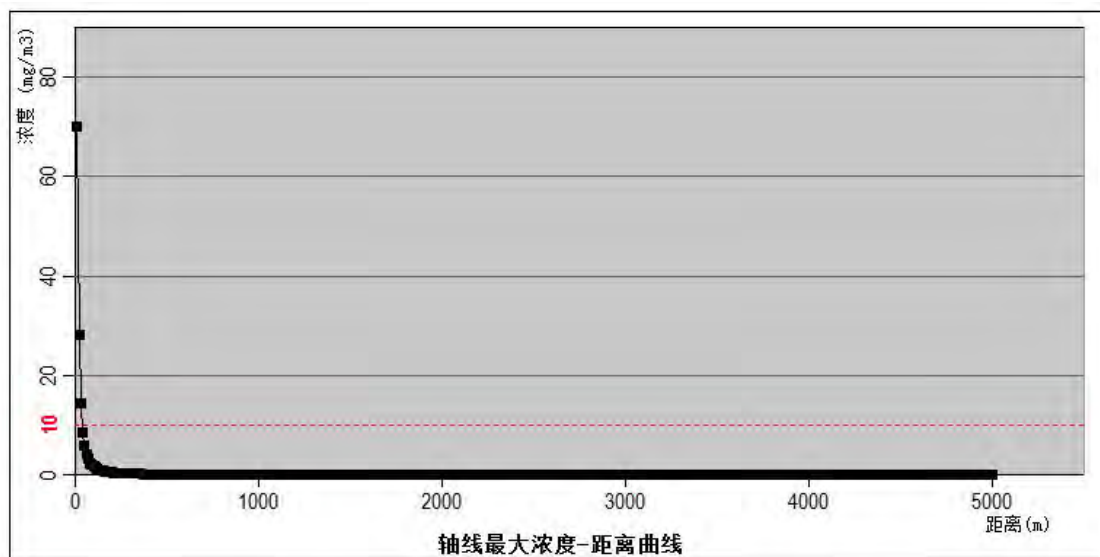
图 6.7-4 最不利气象条件下丁醇轴线最大浓度-距离曲线
