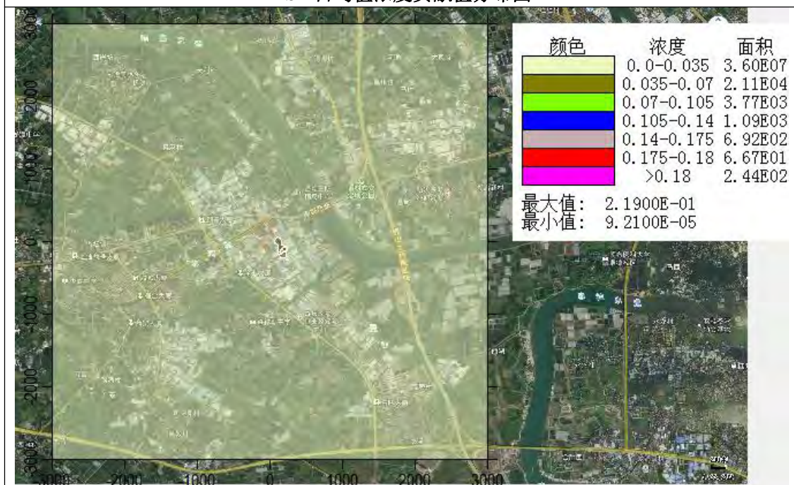
TSP年均浓度贡献值分布图
