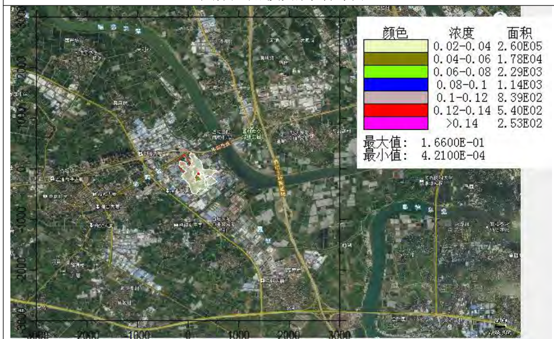
硫酸日均值浓度贡献值分布图
