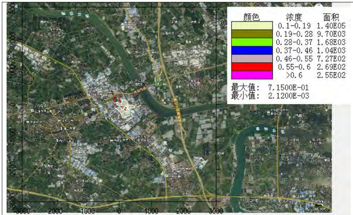
TSP日均值浓度贡献值分布图
