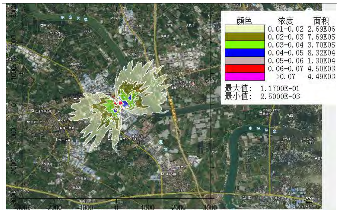
叠加现状浓度后的硫酸小时浓度分布图
