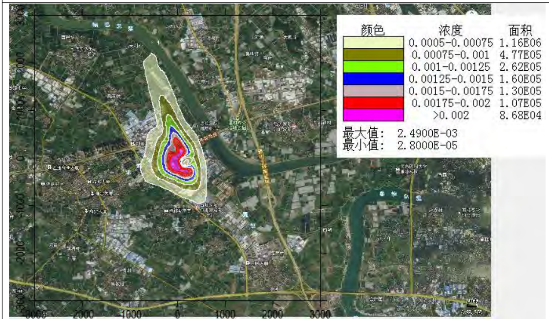
PM 10 年均浓度贡献值分布图
