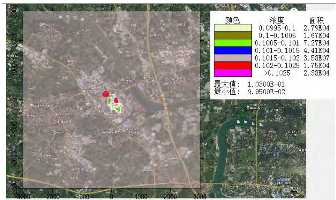
叠加现状浓度后的 PM 10 95% 日均浓度分布图
