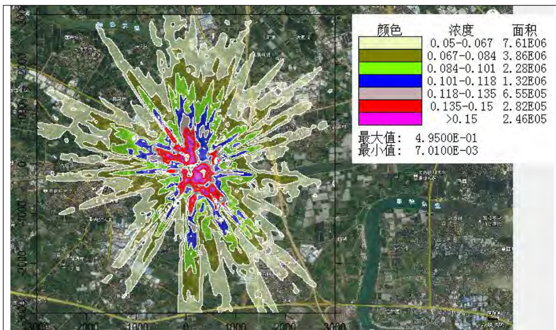
硫酸小时浓度贡献值分布图
