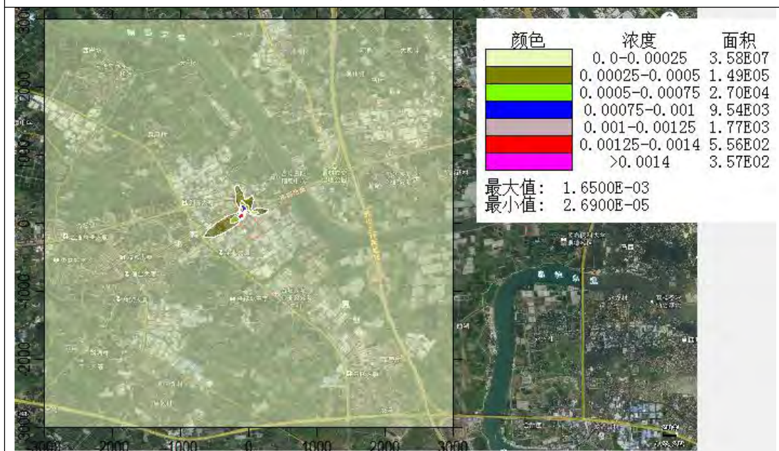
叠加现状浓度后的锡小时浓度分布图
