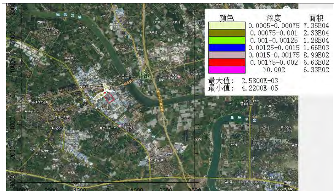
锡小时值浓度贡献值分布图
